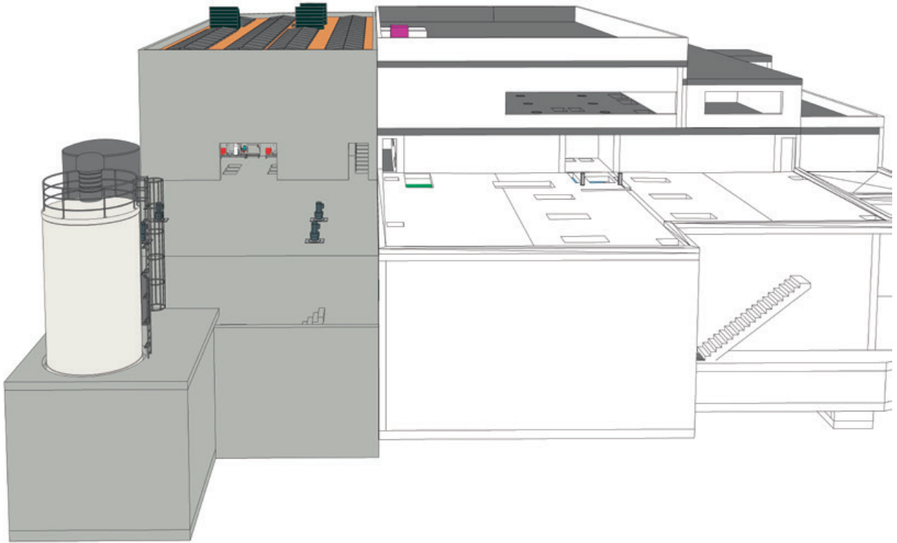
Abbildung 2: 3D-Modell Erweiterung ARA Rorguet (dunkelgraue Bauteile)
