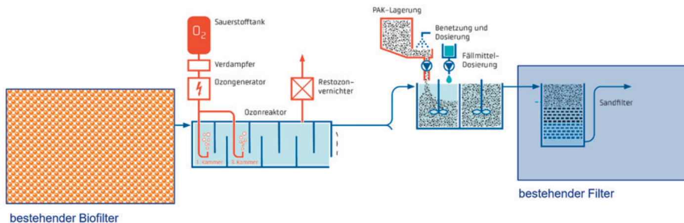
Abbildung 4: Ozonung + PAK-Dosierung + nachgeschaltete Sandfiltration als 4. Reinigungsstufe
